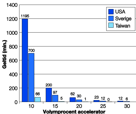
Figur 1: Justerbare geltider med varierende dosering av akselerator. Oppgitte verdier ved 8 °C.
