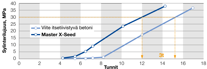
Lujuudenkehitys ajan kuluessa
