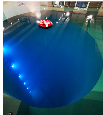
Vista del proceso de ejecución de los trabajos de impermeabilización y acabado de la sima y del vaso y playa de acceso
