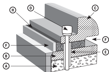
Figure 5 - Application typique d'une cale en résine époxy
