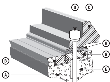
Figure 3 - Traverse ou sole
