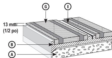
Figure 4 - Traverse typique avec section de joint de dilatation
